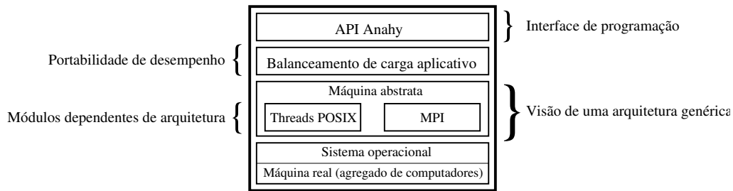
Figura 1: Esquema estruturado do ambiente de programação Anahy
