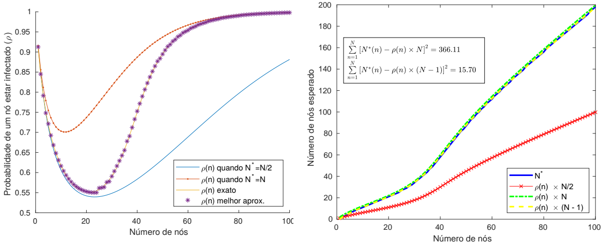
(a) \rho(n) exato e usando aproximações para N^*
