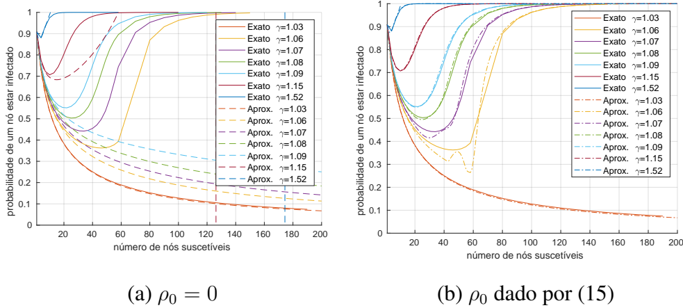
Figura 2. Probabilidade de infecção, calculada usando método de Newton com (a) condição inicial \rho_0 = 0 e (b) heurística para condição inicial.
