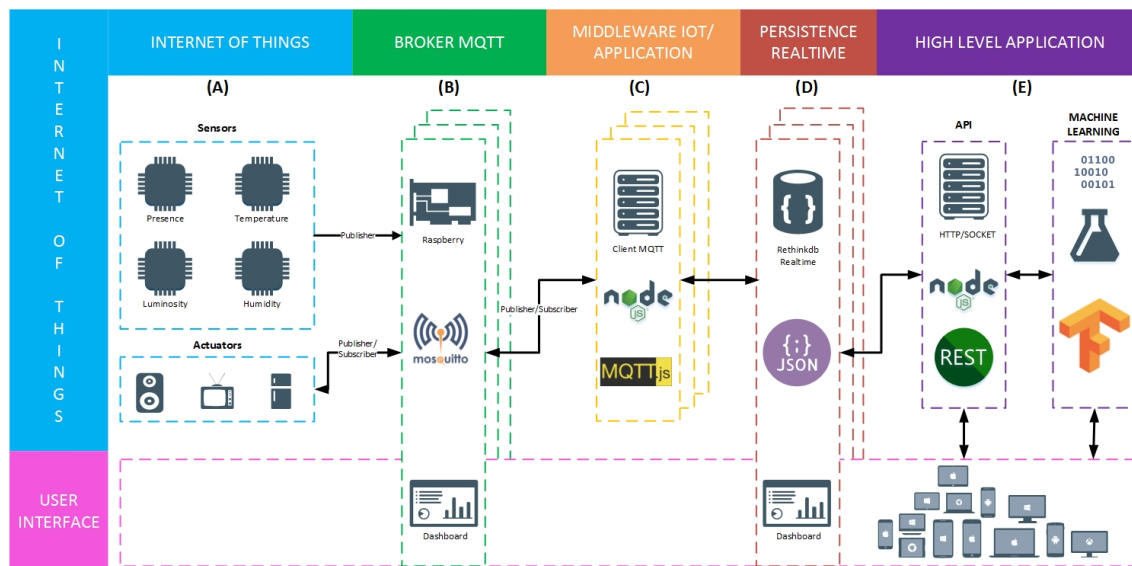
Figura 1. Modelo de arquitetura proposta para a criação da rede de sensores IoT
