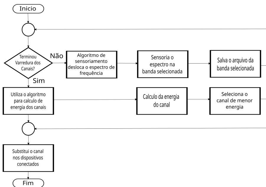
Figura 5. Fluxograma completo do sistema.
