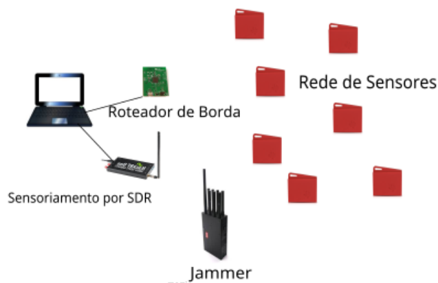
Figura 3. Exemplo de uma Rede de Sensores controlada pelo Sistema de Sensoriamento
