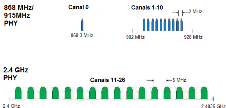
Figura 1. Espectro de radiofrequência IEEE 802.15.4 [Ergen 2004].
