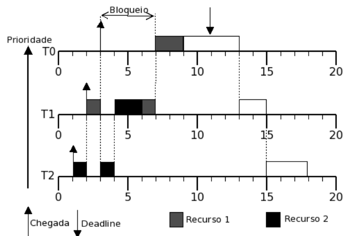
Figura 3. Inversão de prioridade não resolvida por PI
