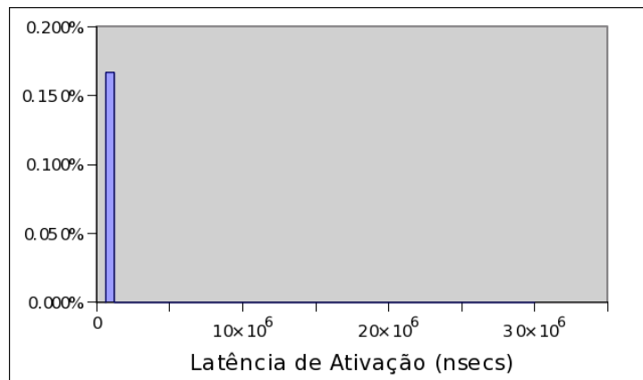
Figura 6. Histograma das latências de ativação (alta prioridade utilizando PI)
