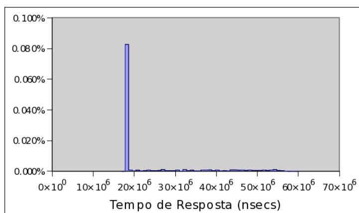
Figura 8. Histograma do tempo de resposta (alta prioridade utilizando PI)
