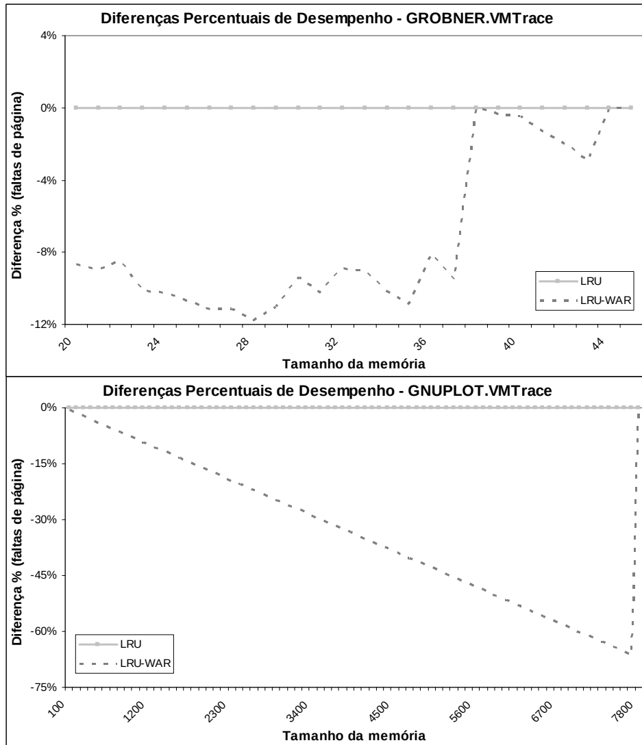
Figura 3. Variação de desempenho do algoritmo LRU-WAR em relação ao LRU
