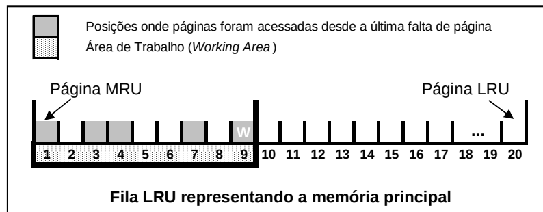
Figura 1. Exemplo de área de trabalho, identificando-se o limite W entre duas faltas de página consecutivas
