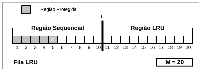
Figura 2. Divisão lógica da fila LRU utilizada pelo algoritmo LRU-WAR
