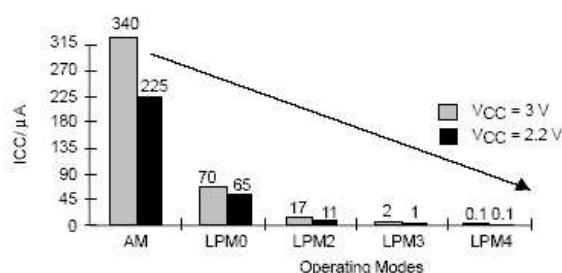
Figura 3: Consumo de corrente nos diferentes modos de operação.
