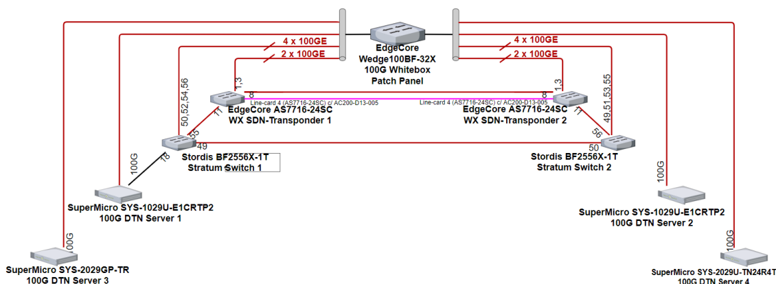
Figura 1. Equipamentos e conexões implementadas no Lab. SDN Multicamadas.
