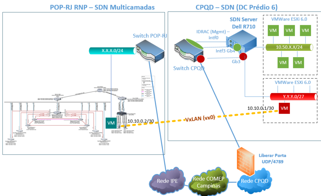
Figura 3. Topologia de interconexão entre o CPQD e o testbed SDN Multicamadas.
