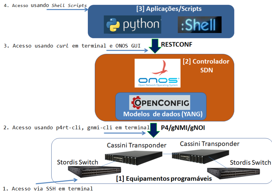
Figura 4. Arquitetura de camadas empregada nos testes propostos.
