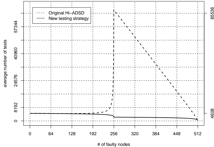
Figura 3. Número de testes médio em uma rede estável de 512 nodos no pior caso do algoritmo Hi-ADSD .
