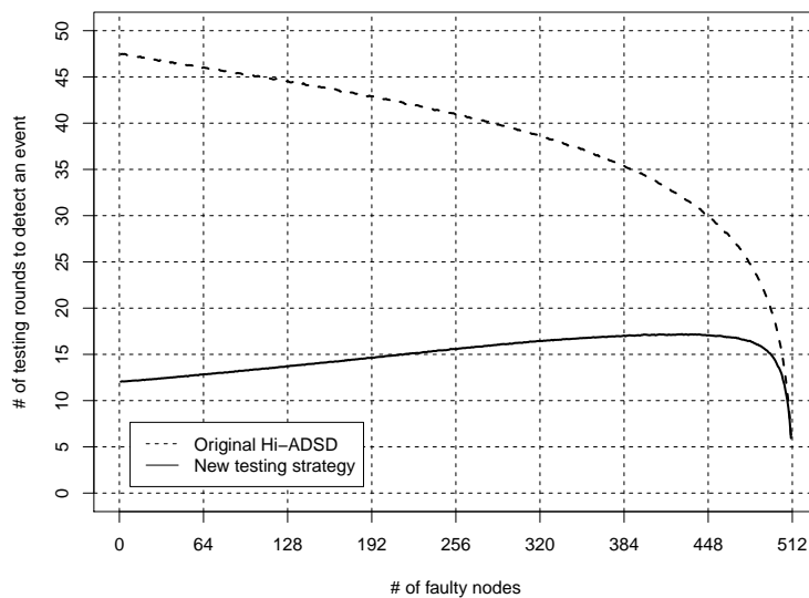
Figura 6. Latência média para detecção de um evento em uma rede de 512 nós.
