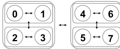
Figura 2. Clusters formados pelo algoritmo Hi-ADSD em um sistema de 8 nodos.
