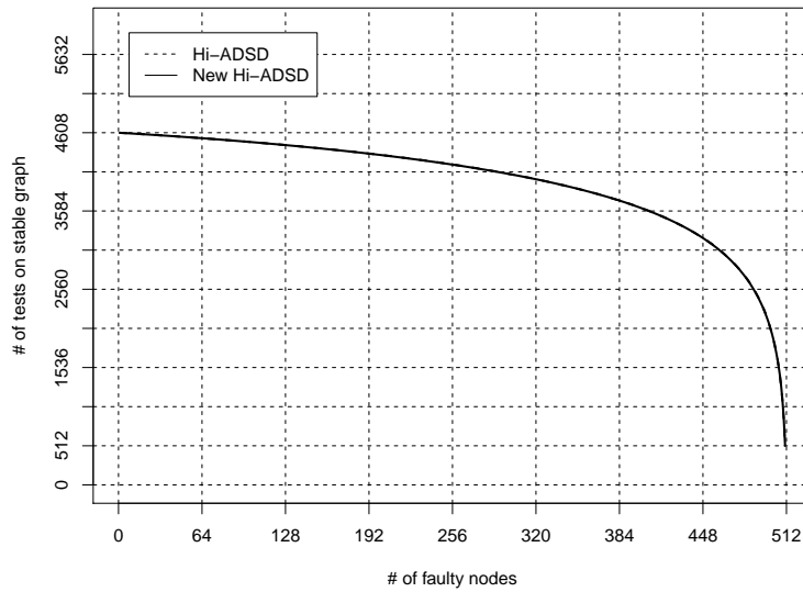
Figura 5. Número de testes médio em uma rede estável de 512 nós.
