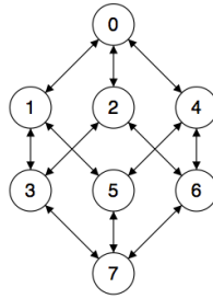
Figura 1. Um 3-hipercubo.
