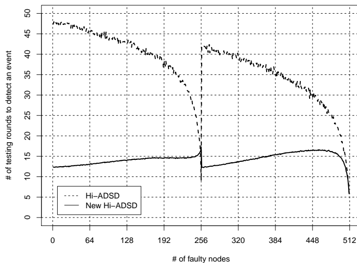
Figura 4. Latência média para detecção de um evento em uma rede de 512 nodos no pior caso do algoritmo Hi-ADSD .
