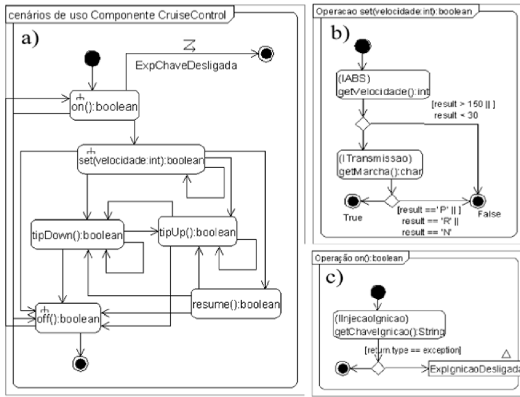
Figura 1 (a) DCU do componente CruiseControl; (b) DIOs das Operações set e; (c) on
